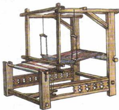
Ткацкий станок. Реконструкция Б. Колчина
